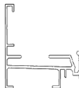
Профиль нижний для 40-S мм арт. 420031
