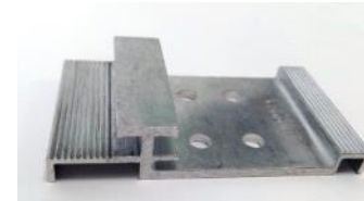
Анкер для 40-5 мм арт. 49404050
