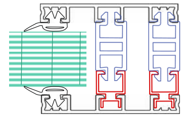
Уплотнитель ТЭП арт. 902904
